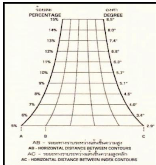
ภาพที่ 3.16 คำแนะนำเกี่ยวกับความลาดชัน
