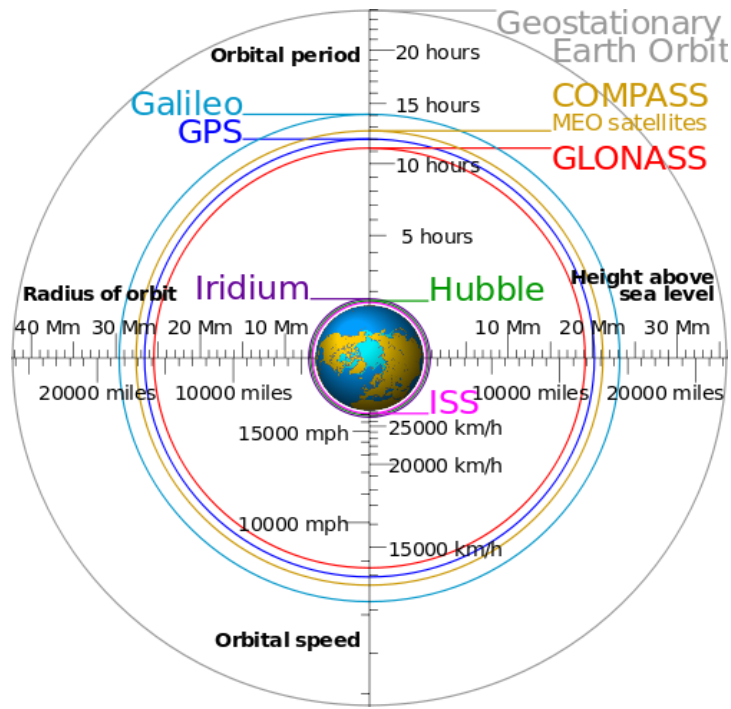
ภาพที่ 8.6 ระยะเวลาโคจรและความสูงของดาวเทียมระบบกำหนดตำแหน่งบนพื้นโลกภาคพื้น (แหล่งที่มา: https://www.masterclock.com/company/masterclock-inc-blog/ )
