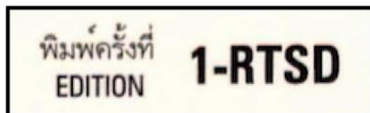
ภาพที่ 3.6 หมายเลขการจัดพิมพ์และหน่วยงานที่จัดพิมพ์
