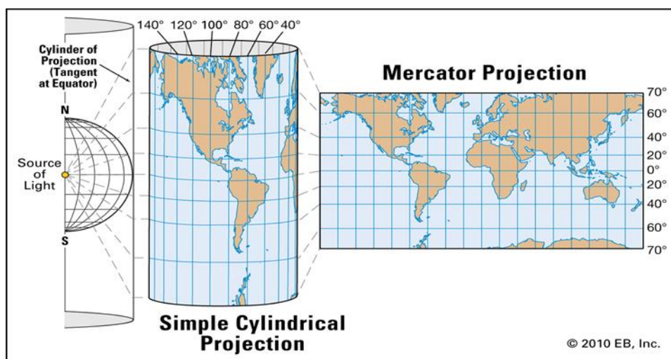
ภาพที่ 1.6 แผนที่โลกจากการฉายภาพโลกลงบนแผ่นวัสดุทรงกระบอก
