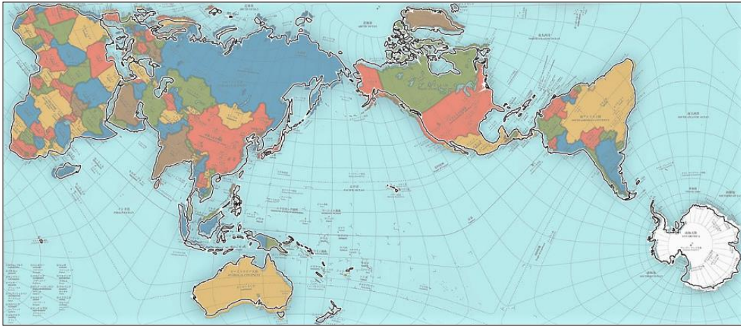
ภาพที่ 2.16 โครงแผนที่ AuthaGraph ที่มีขนาดของพื้นที่ความถูกต้องมากที่สุดในปัจจุบัน
