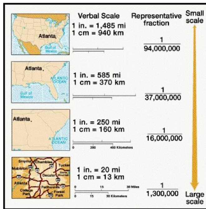
ภาพที่ 1.11 มาตราส่วนแผนที่จากมาตราส่วนเล็ก (บน) ไปยังมาตราส่วนใหญ่ (ล่าง) (แหล่งที่มา : https://mygeoskills.wordpress.com/maps/structure/scale-of-a-map/ )
