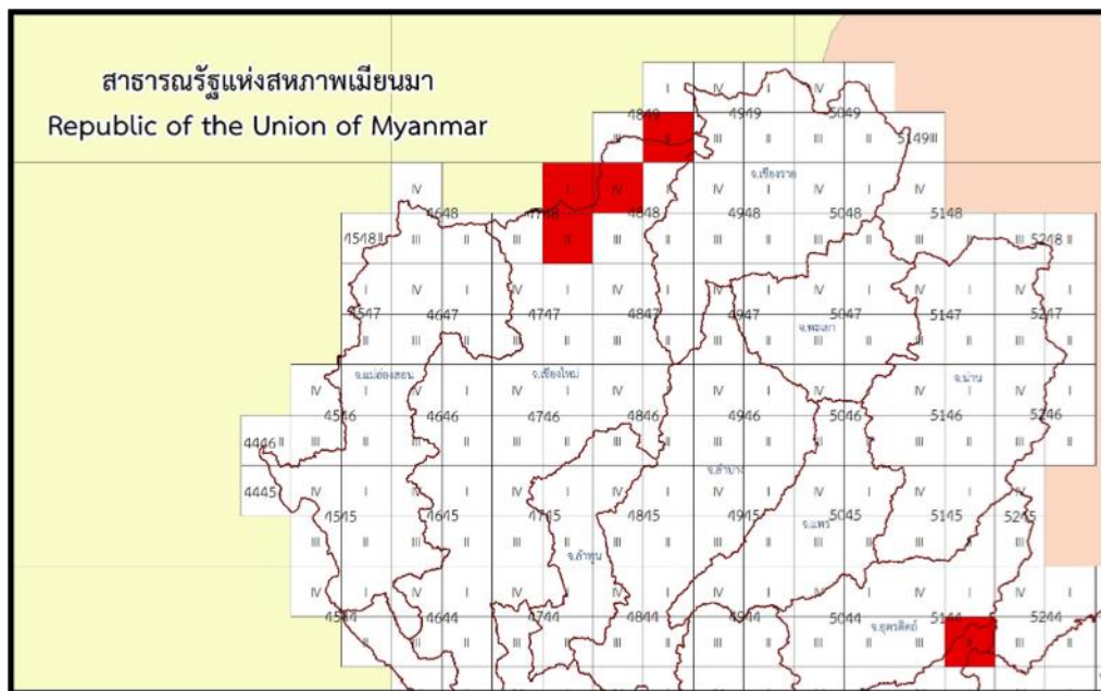
ภาพที่ 3.4 การเรียงลำดับหมายเลขระวางแผนที่
