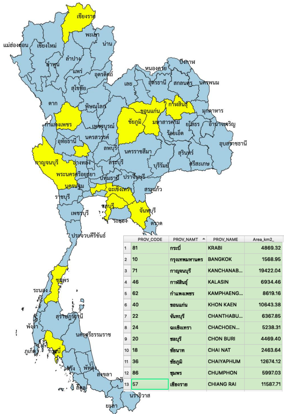
ภาพที่ 5.15 ผลจากการหาขนาดพื้นที่ด้วยโปรแกรมเฉพาะทางบนโปรแกรม QGIS 3.6 (แหล่งที่มา: จัดทำโดยผู้เขียน)
