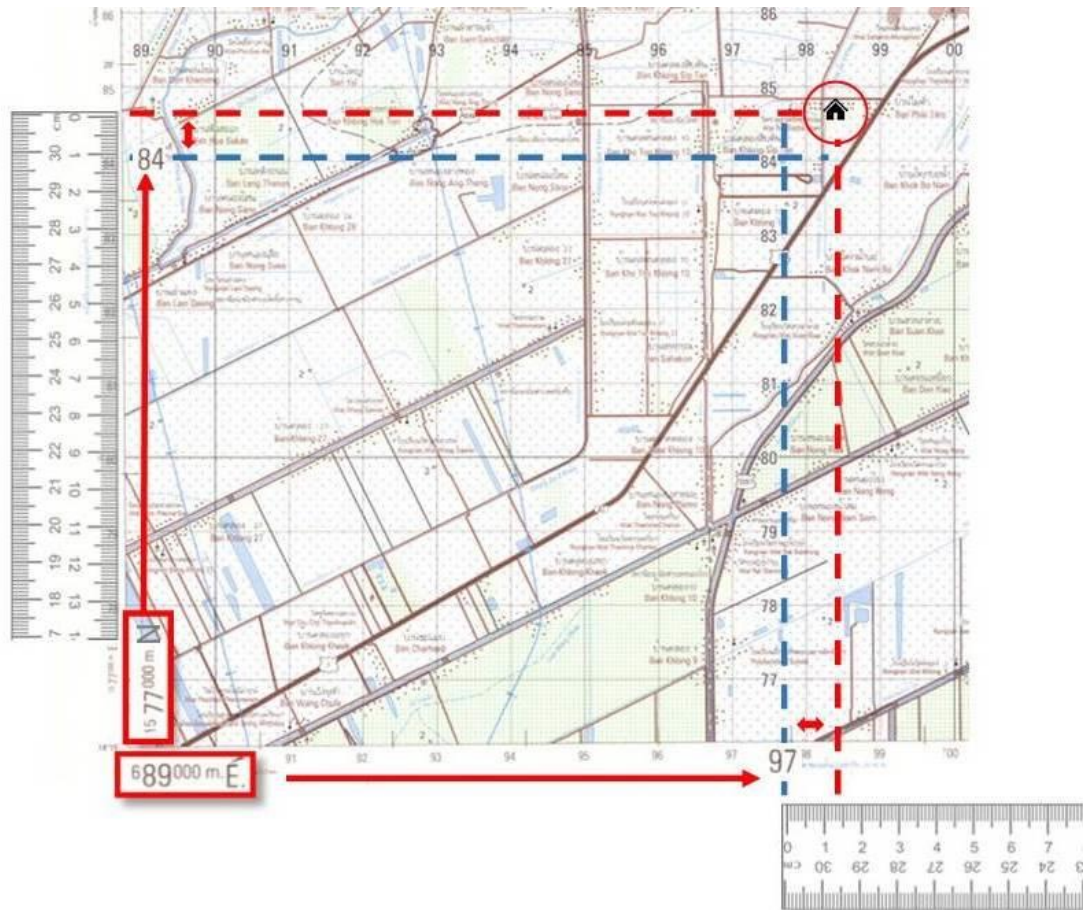
ภาพที่ 3.19 การกำหนดตำแหน่งพิกัดกริด (แหล่งที่มา: จัดทำโดยผู้เขียน)
