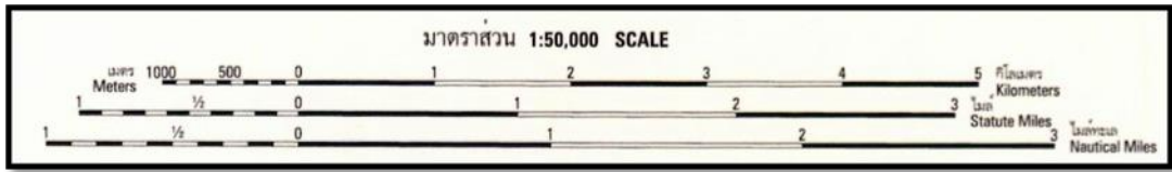
ภาพที่ 3.7 มาตราส่วนแบบสัดส่วนและมาตราส่วนบรรทัด
