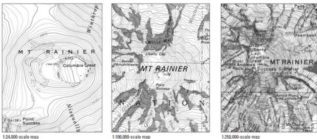
ภาพที่ 4.10 การเปรียบเทียบแผนที่ที่มีมาตราส่วนต่างกัน
