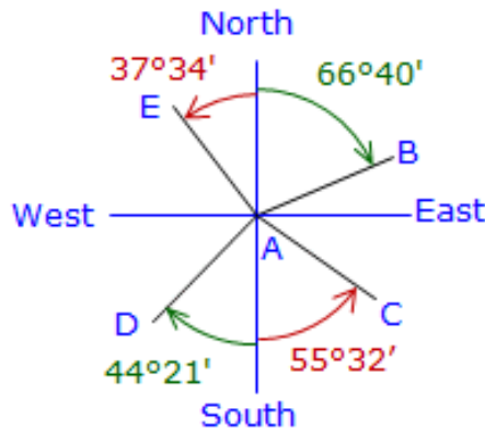
ภาพที่ 4.6 การบอกทิศตามค่ามุมแบริ่ง
