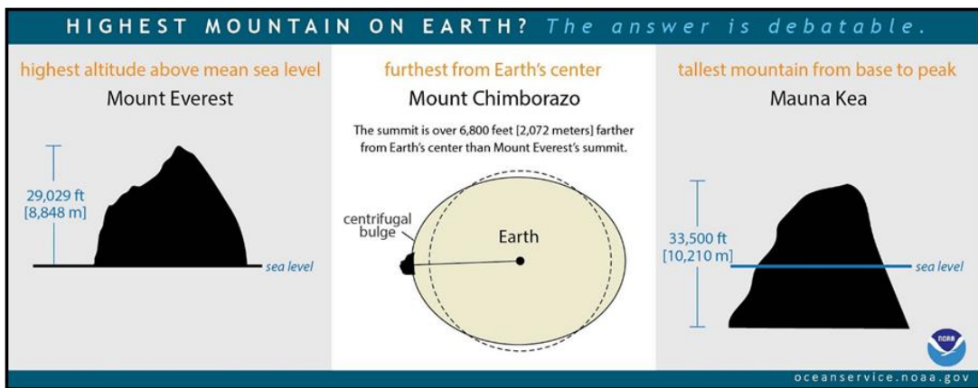
ภาพที่ 2.6 เกณฑ์ที่ใช้ในการวัดความสูงของจุดที่สูงที่สุดบนโลกทั้ง 3 เกณฑ์ (แหล่งที่มา: https://oceanservice.noaa.gov/facts/highestpoint.html )
