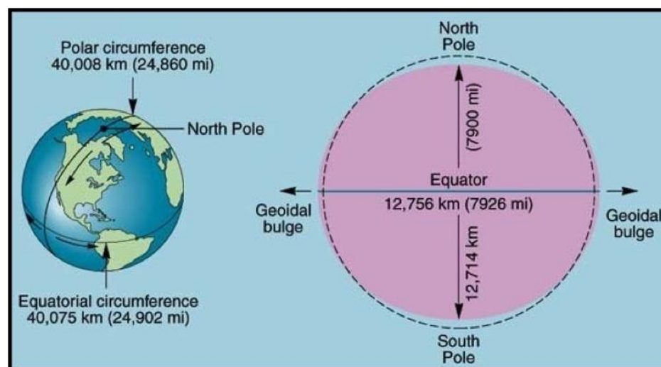
ภาพที่ 2.4 เส้นผ่าศูนย์กลางของโลกที่ต่างกันจากรูปทรงสัญญาณที่เป็นทรงรี
