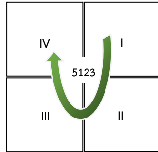
ภาพที่ 3.3 หมายเลขระวางแผนที่และทิศทางการอ่านระวาง
